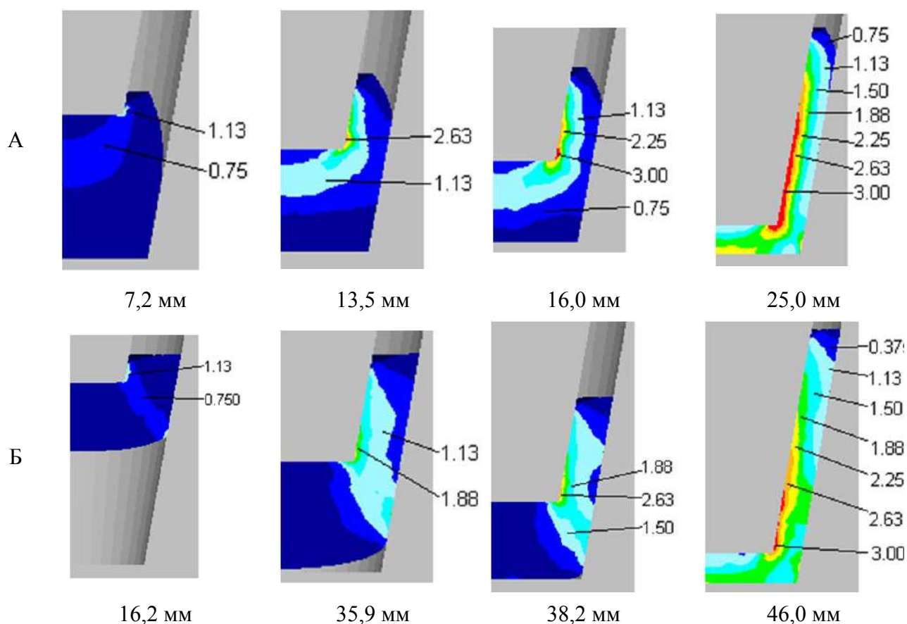
Рис. 7. Розподіл інтенсивності деформації \varepsilon_i за перетином заготовки по ходу процесу (в мм) при зворотному (А) і комбінованому видавлюванні (Б)
